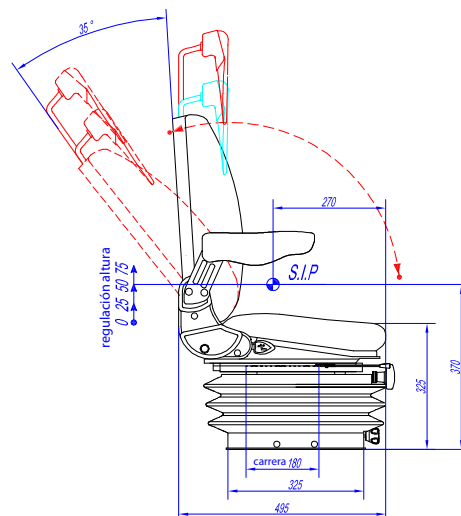
RM92210 Ref.: 0192237G2020 Suspensión neumática Pneumatic suspension
