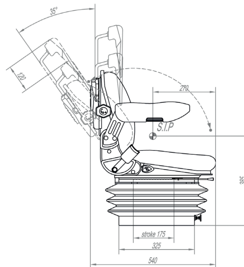
RM62210 Ref: 010623752020 Suspensión mecánica Mechanical suspension
